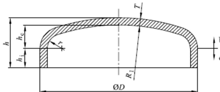
Rys. 1 Dno koszykowe
