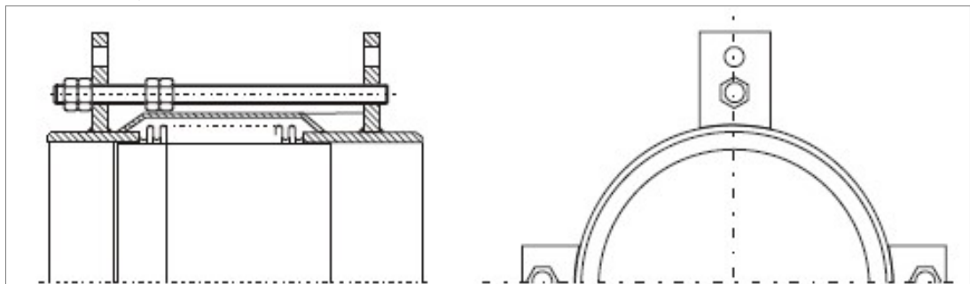
Rysunek 10. Pojedynczy mieszkowy kompensator osiowy przeznaczony do montażu w komorze ciepłowniczej
