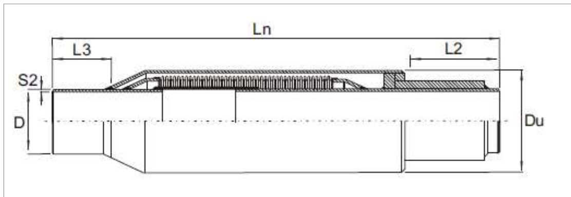
Rysunek 12. Mieszkowy kompensator osiowy przeznaczony do preizolacji
