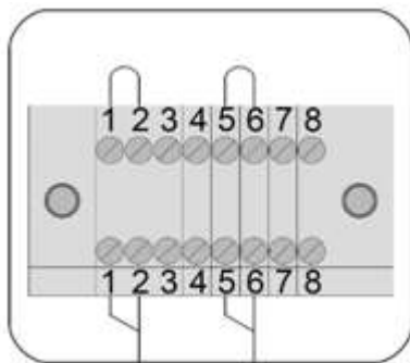
Rys. 9 Łączenie przewodów kontrolnych z przewodem dwużyłowym oraz wyprowadzenie przewodu po stronie rury wewnętrznej
