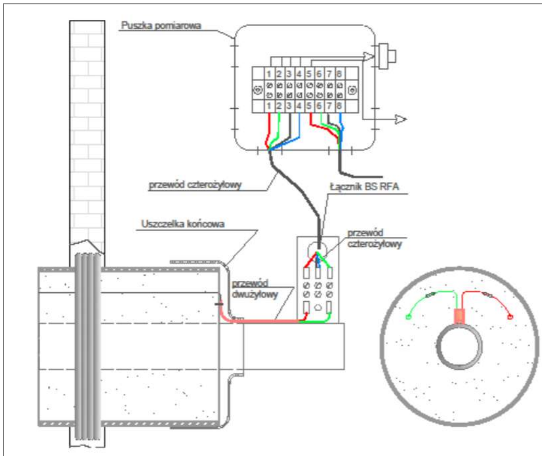
Rys. 13 b Połączenie przewodów instalacji alarmowej z puszką pomiarową
