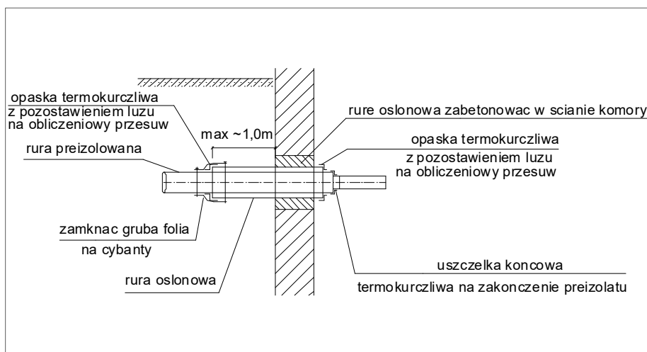
Rysunek 3a. Schemat przykładowego rozwiązania przy przejściu rurociągu preizolowanego w rurze ochronnej przez ścianę komory
