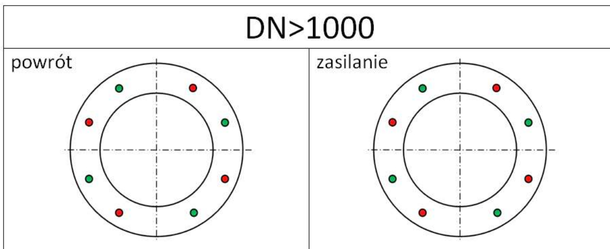
Rysunek 3b. Rozmieszczenie przewodów systemu nadzoru (patrząc od źródła ciepła) w rurach preizolowanych > DN 1000
