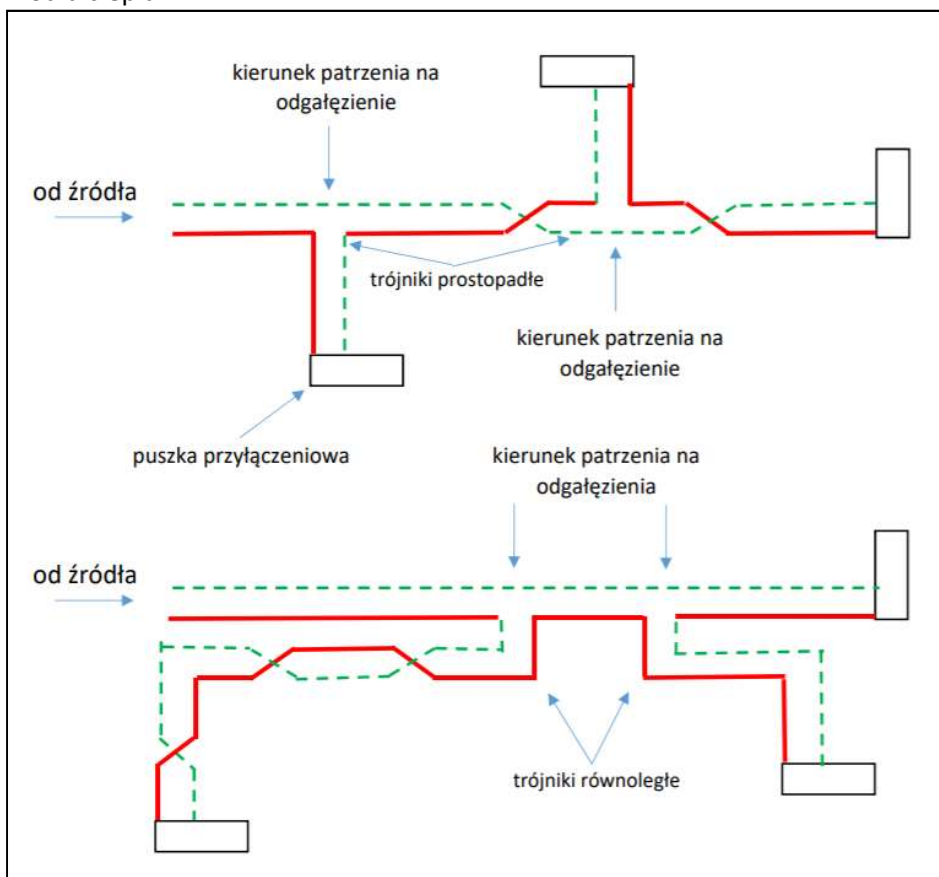
Rys. 17 Reguła prawostronności
