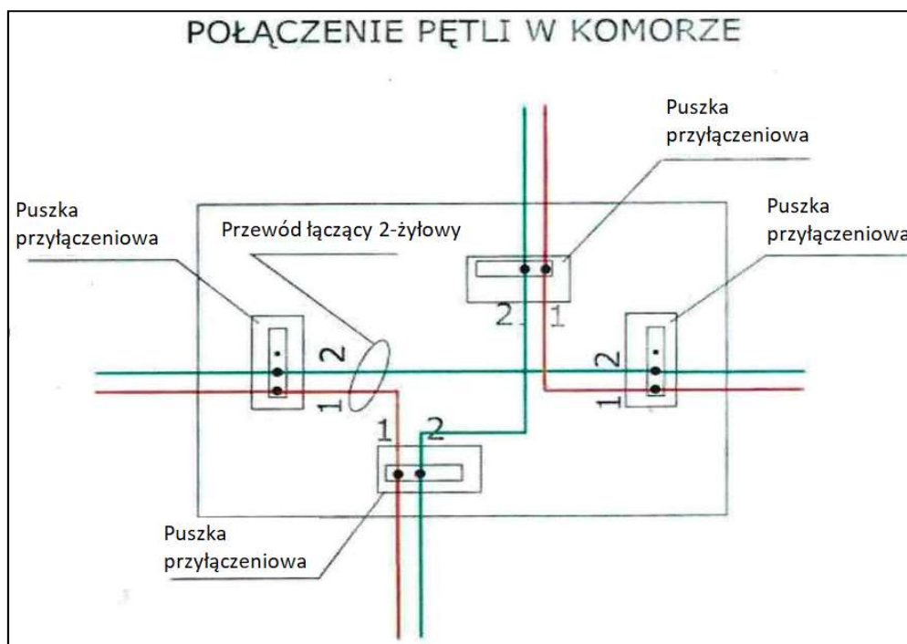
Rysunek 21 Schemat okablowania rozgałęzień
