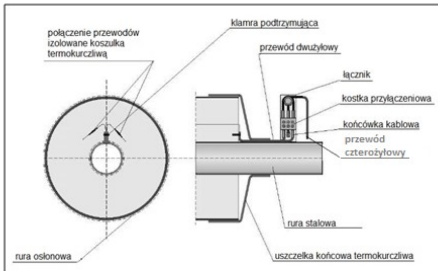
Rys. 13 a Połączenie przewodów instalacji alarmowej z łącznikiem
