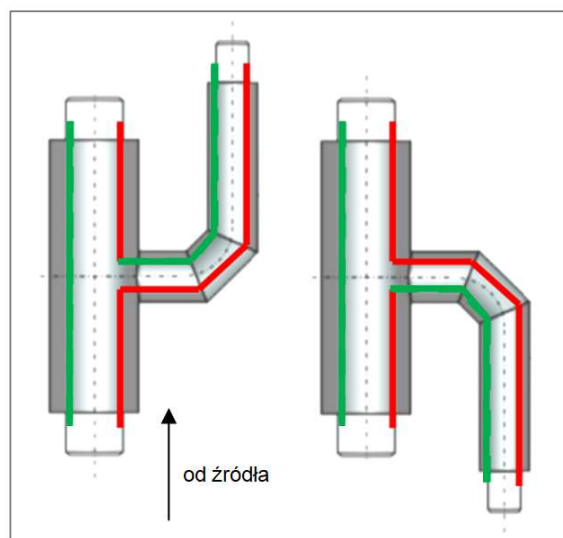
Rys. 14, 15a, 15b, 16a, 16b Schematy przewodowania łuków, odgałęzień prostopadłych i równoległych
