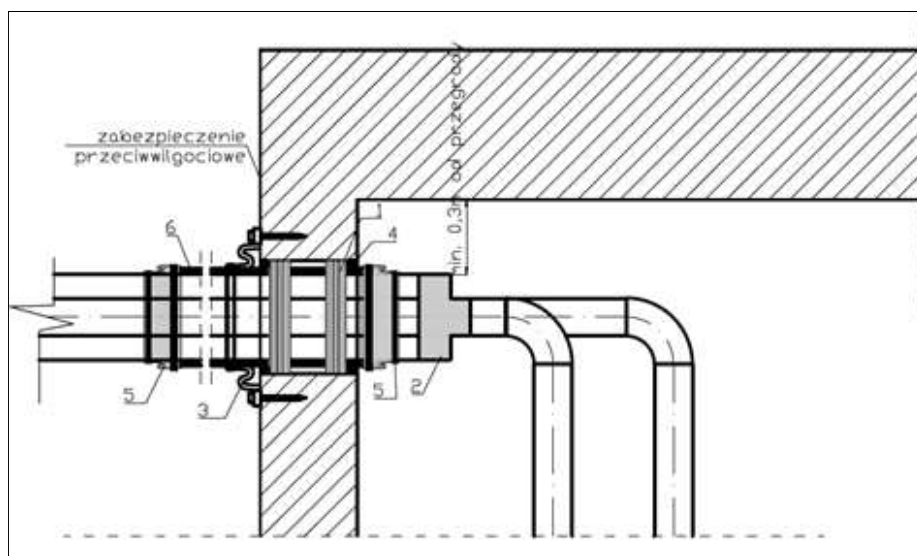
Rysunek 3c. Schemat przykładowego rozwiązania przy przejściu rurociągu preizolowanego w rurze ochronnej przez ścianę zewnętrzną budynku
