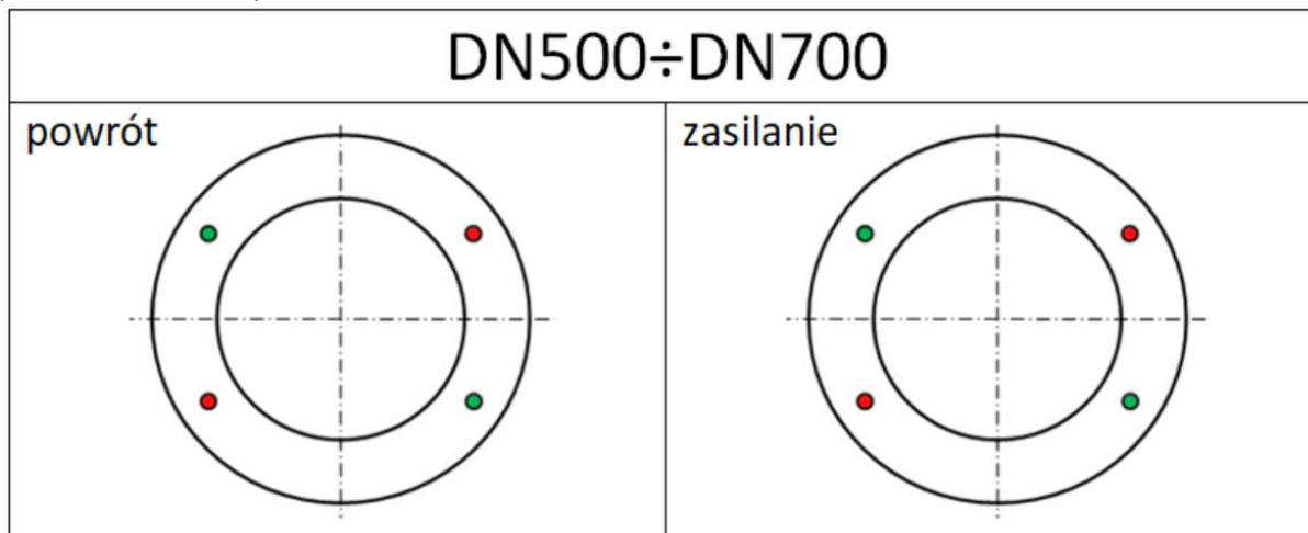
Rysunek 2. Rozmieszczenie przewodów systemu nadzoru (patrząc od źródła ciepła) w rurach preizolowanych 500 \leq DN \leq 700
