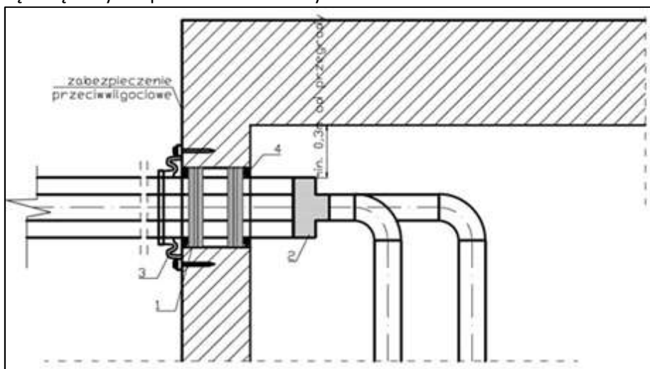
Rysunek 3b. Schemat przykładowego rozwiązania przy przejściu rurociągu preizolowanego przez ścianę zewnętrzną budynku
