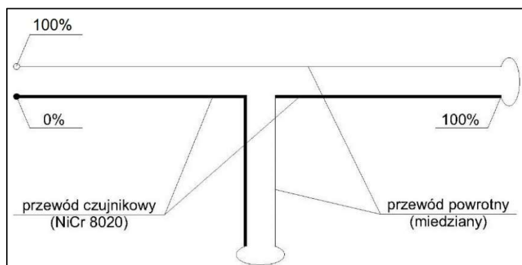
Rys. 5 Pętla pomiarowa z odgałęzieniem prostopadłym
