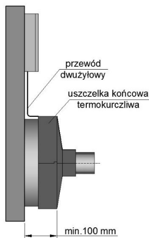
Rys. 11 Wyprowadzenie i zamknięcie pętli w puszcze przyłączeniowej
