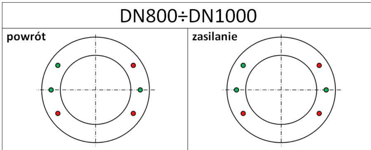
Rysunek 3a. Rozmieszczenie przewodów systemu nadzoru (patrząc od źródła ciepła) w rurach preizolowanych DN 800 ÷ DN 1000
